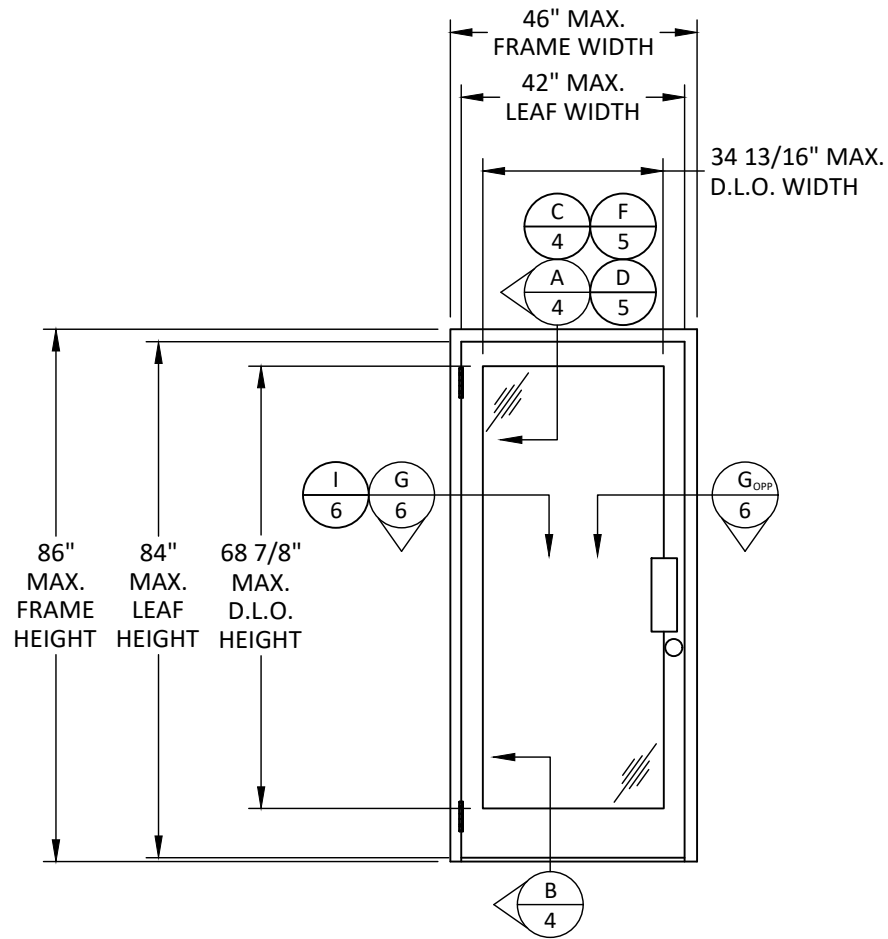
ELEVATION
