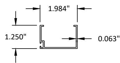
36 OHCC DOOR STOP
