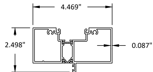
8 TRANSOM BAR
