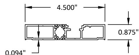
33 THERMAL JAMB SUBFRAME (FLAT)
