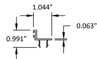
35 DOOR STOP
