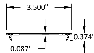
28 FILLER
